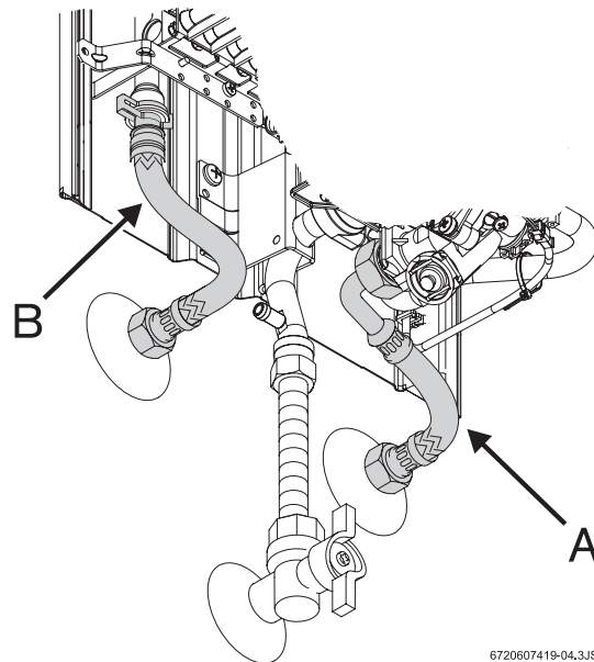
Рис. 5 Підключення до водопроводу
