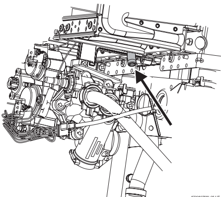
Рис. 13 Контрольна точка вимірювання тиску
