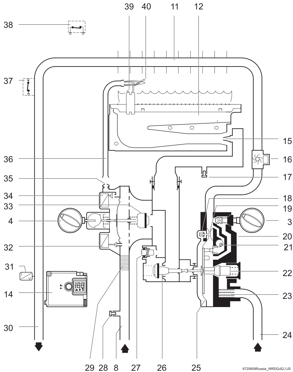
Рис. 2 Схема пристрою
