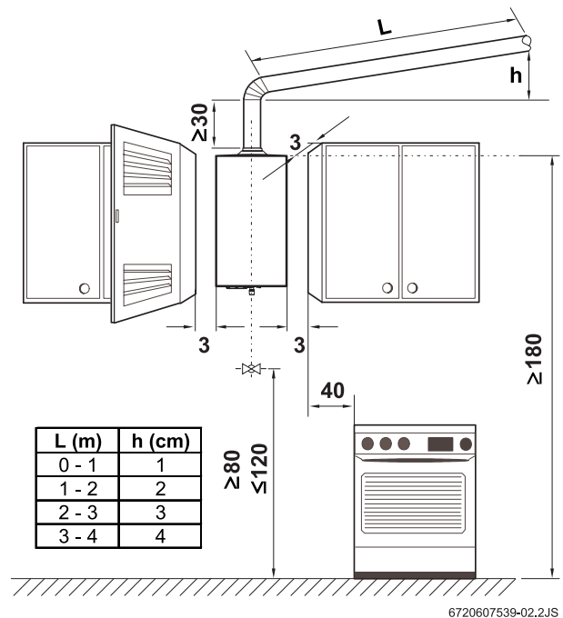
Рис. 4 Мінімальні допуски
