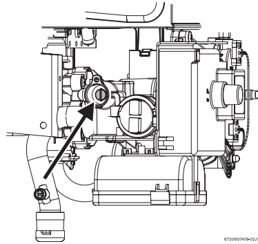
Рис. 14 Гвинт регулювання максимального тиску газу
