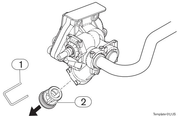
Рис. 15 Злив води
