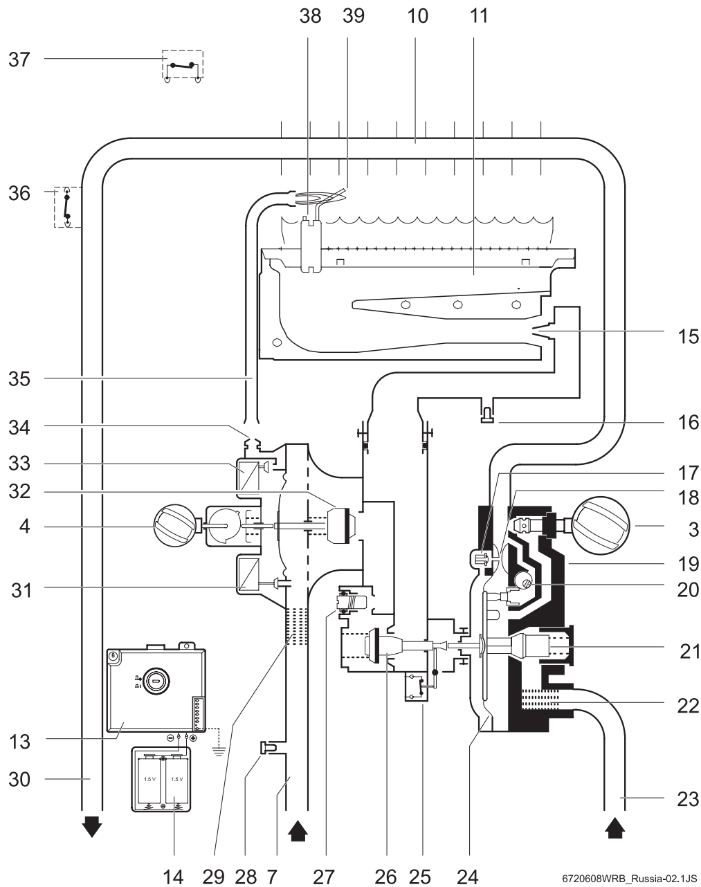
Рис. 2 Функціональна схема
