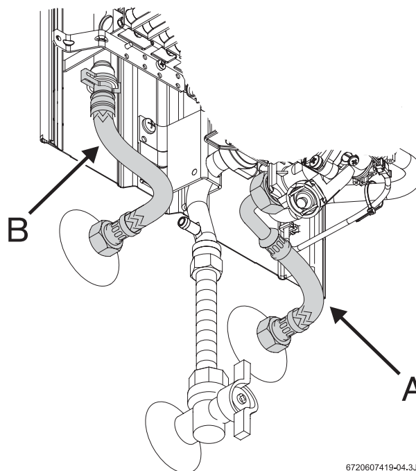
Рис. 5 Підключення до водопроводу
