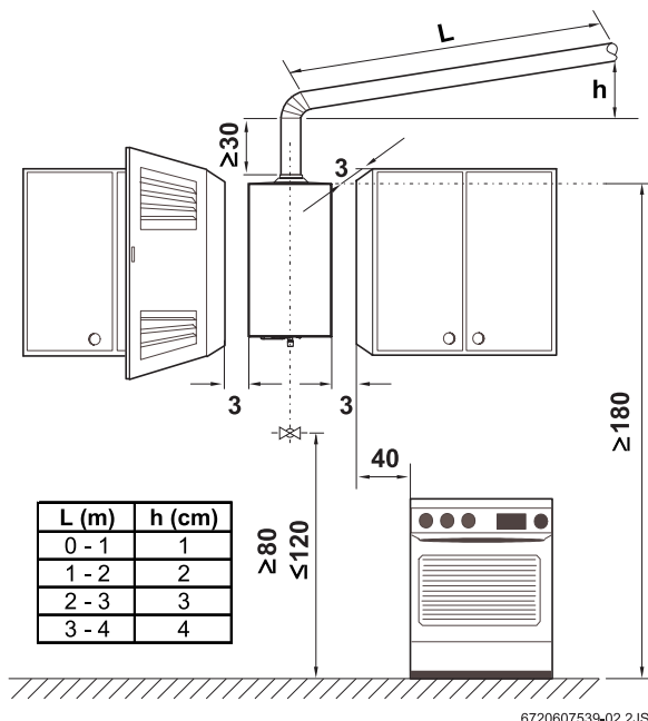
Рис. 4 Мінімальні допуски
