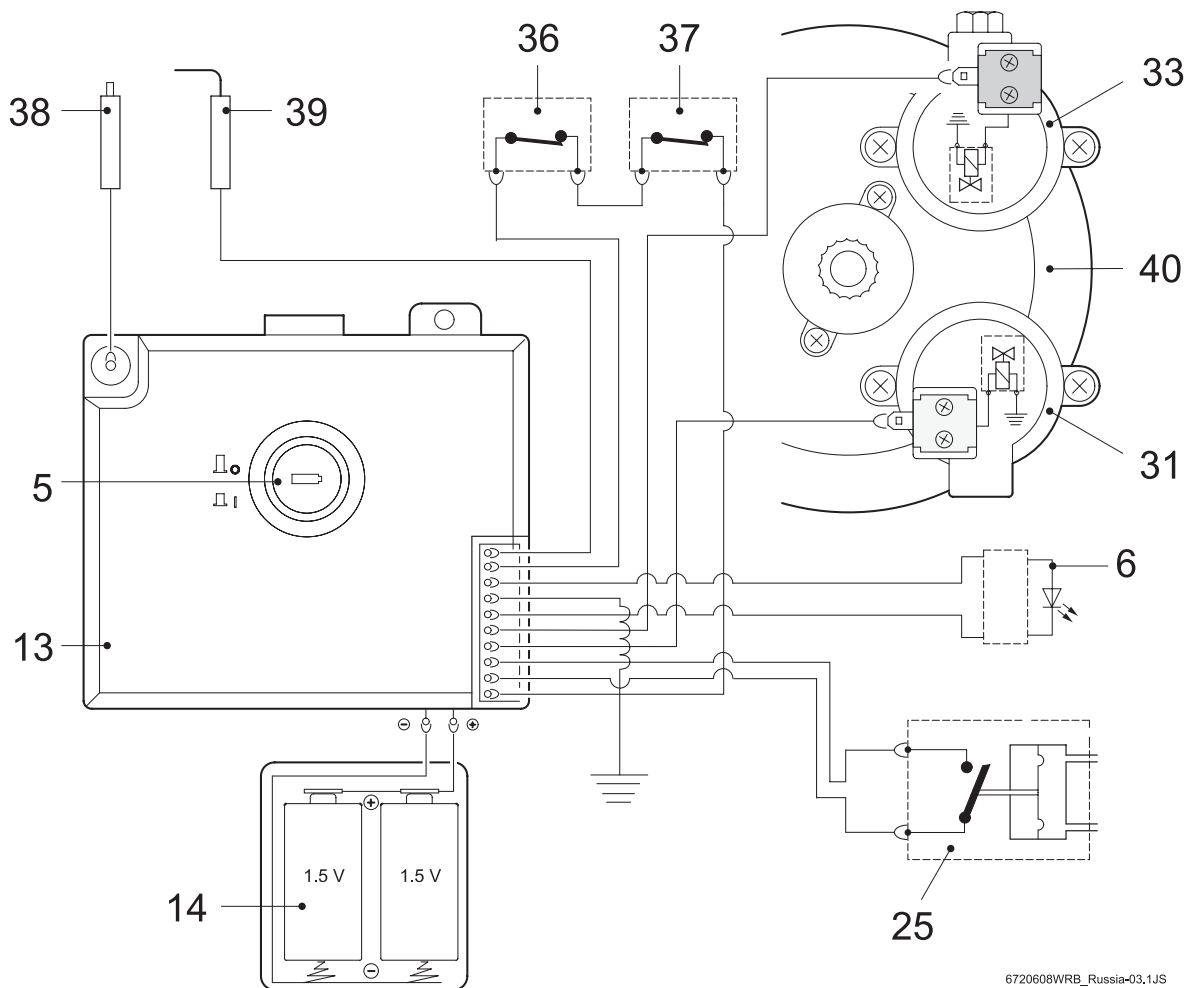
Рис. 3 Електрична схема
